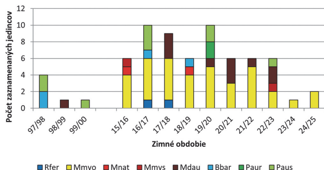
Obr. 25. Počty jedincov jednotlivých druhov netopierov (okrem Rhinolophus hipposideros ) zaznamenaných v jaskyni Pec počas sledovaných zimných období.
