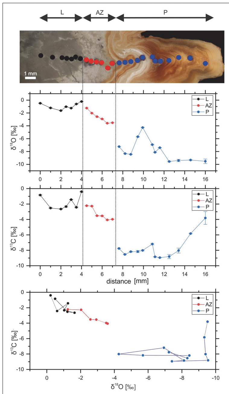
Obr. 6. Zloženie stabilných izotopov vápenca a kalcitového hráškovitého sintra na stene jaskyne spodnej vývojovej úrovne Plaveckej jaskyne: L – neporušený (nezmenený) vápenec, AZ – alterovaná zóna zmeny v najvrchnejšej časti vápenca, P – kalcitový hráškovitý sinter (Bella et al., 2019b).
