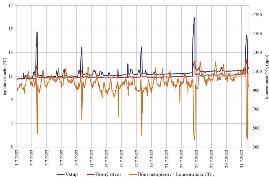
Obr. 13. Hodinové hodnoty koncentrácie \text{CO}_2 v Dóme netopierov v porovnaní s teplotou vzduchu vo Vstupe a Hornom otvore . Fig. 13. Hourly \text{CO}_2 concentrations in the Bat Dome , compared to air temperatures in the Entrance and Upper opening .
