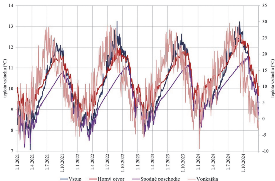
Obr. 10. Priemerné denné teploty vzduchu v dynamickej časti jaskyne a na vonkajšej stanici.
