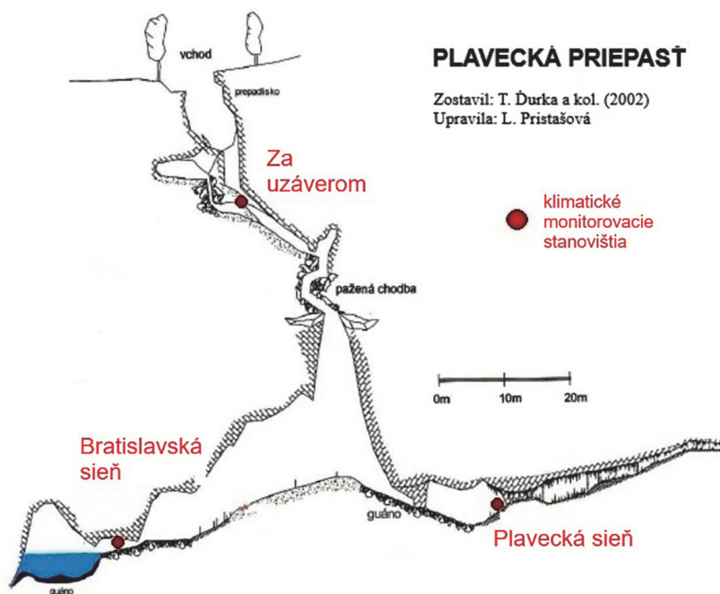
Obr. 3. Bočný rez Plaveckej priepasti, lokalizácia meracích stanovišť.
