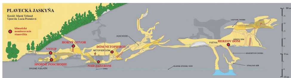
Obr. 5. Bočný rez Plaveckej jaskyne, lokalizácia meracích stanovišť. Fig. 5. Side view of the Plavecká Cave, location of measurement sites.
