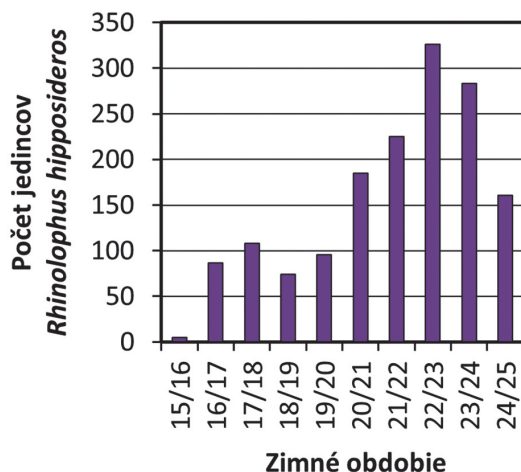
Obr. 24. Počty hibernujúcich jedincov druhu Rhinolophus hipposideros zaznamenané v jaskyni Pec v zimných obdobiach 2015/2016 až 2024/2025. Fig. 24. Numbers of hibernating individuals of Rhinolophus hipposideros recorded in the Pec Cave in the winter periods 2015/2016 to 2024/2025.
