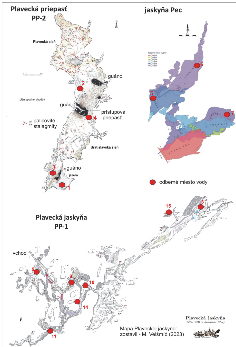
Obr. 2. Mapa Plaveckej jaskyne, Plaveckej priepasti a jaskyne Pec s odbernými miestami vzoriek vôd (upravené podľa Velšmída, 2013; Šmída, 2010).
