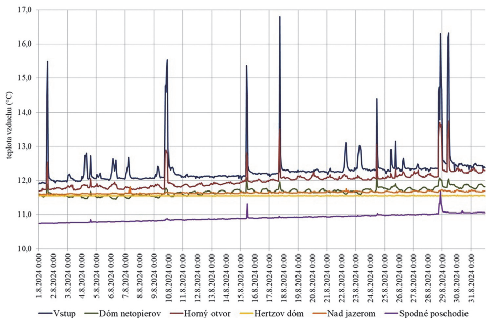
Obr. 12. Hodinové teploty vzduchu na jednotlivých stanovištiach v letných mesiacoch. Fig. 12. Hourly air temperatures at the individual sites during the summer months.
