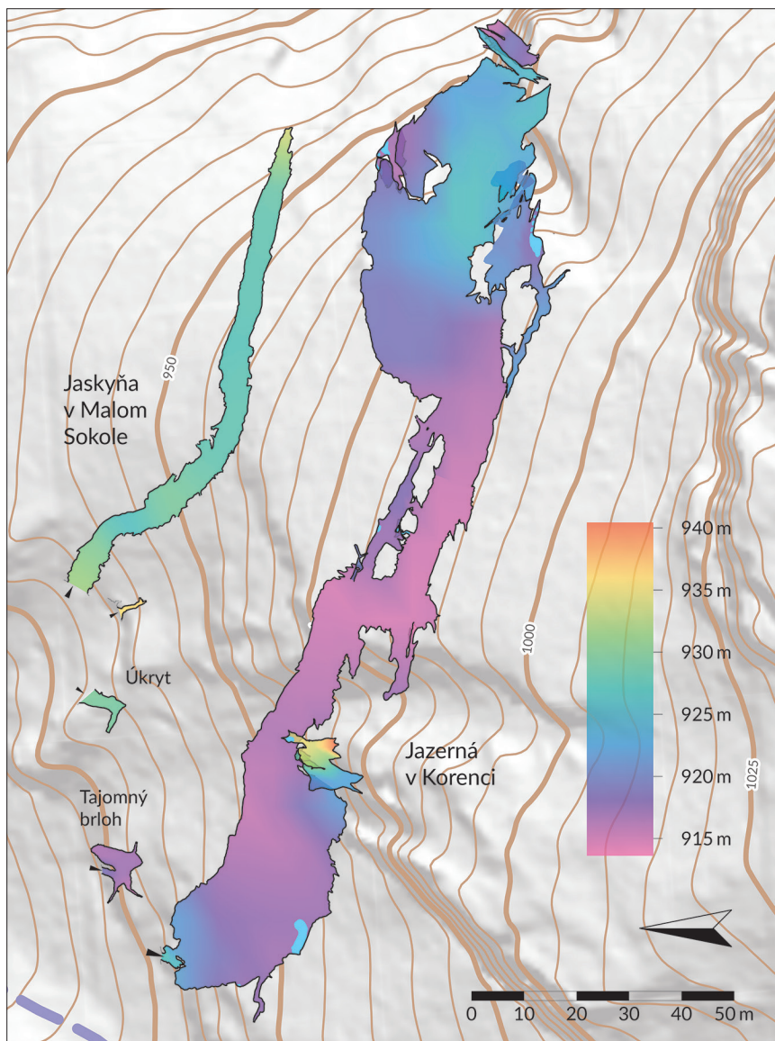
Obr. 5. Jazerná v Korenci a okolité jaskyne. Pôdorys.
