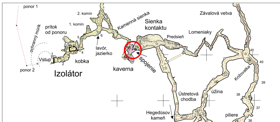
Pôdorys ponoru Izolátor a príľahlej časti Čertovej diery.
