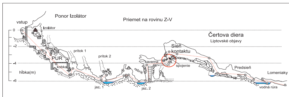
Bokorys ponoru Izolátor a príľahlej časti Čertovej diery.
