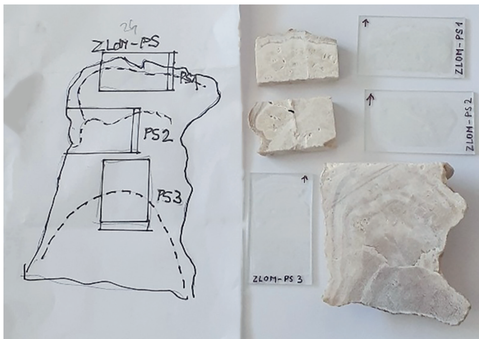
Obr. 6. Príklad rozloženia leštených výbrusov, aby pokryli najdôležitejšie viditeľné miesta zmeny rastu stalagmitu PS.
