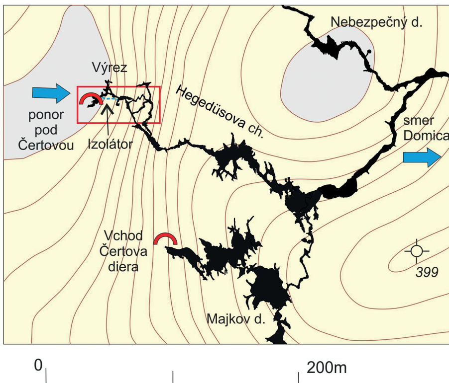
Situačná mapa Čertovej diery a ponoru Izolátor.
