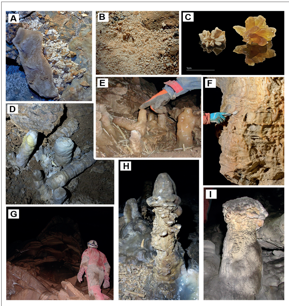
Obr. 2. Kryogénne speleotémy a produkty deštruktívnych procesov súvisiacich so zamŕzaním vody v homotermálnych jaskyniach. A) a B) CCC-c Pilierová sieň Jaskyňa zlomísk, C) detail na agregáty CCC-c z Četnikovej svadby, Strážovské vrchy, D) deštrukcia stalagmitov Jaskyňa zlomísk, E) lámané kvaple Jaskyňa zlomísk, F) ľadové prílepk, Závojová sieň, G) rozlámané masívne kôry homoľového stalagmitu, Stratenský jaskynný systém, H) deformovaný stalagmit PS, I) deformovaný stalagmit, Pustá jaskyňa. Foto: J. Šurka, J. Česla, R. Milovský, M. Orvošová Fig. 2. Cryogenic speleothems and cryogenically induced degradation features related to water freezing in homothermal caves. Cryogenic speleothems: (A–B) Coarse-grained cryogenic cave carbonates (CCC-c), Pillar Hall, Jaskyňa Zlomísk Cave; (C) Detail of CCC-c aggregates from Četnikova Svadba Cave, Strážovské vrchy Mountains. Cryogenic degradation features: (D) Stalagmite degradation, Jaskyňa Zlomísk Cave; (E) Breakdown fragments, Jaskyňa Zlomísk Cave; (F) Ice attachments (ice accretions), Závojová Hall; (G) Fragmented massive crusts of a “mound-shaped” stalagmite, Stratenská Cave system; (H) Deformed stalagmite, PS Dóm, Zlomísk Cave; (I) Deformed stalagmite, Pustá Cave. Photo: J. Šurka, J. Česla, R. Milovský, M. Orvošová
