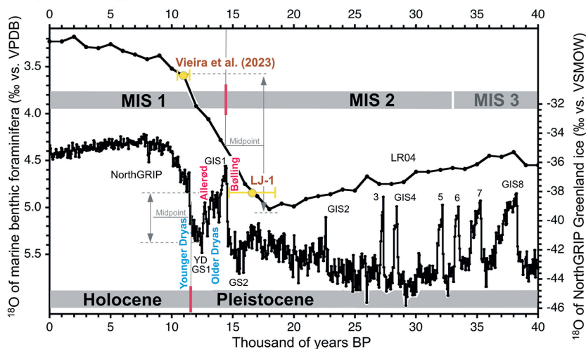
Obr. 4. Vek datovaných travertínov z Liptovského Jána, znázornený v schéme B. Railsbacka z roku 2017.
