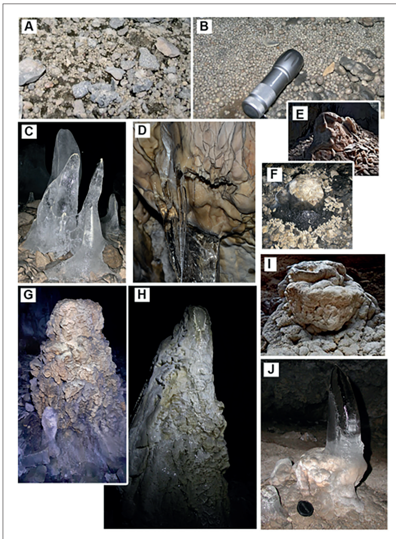
Obr. 1. Kryogénne speleotémy a produkty deštruktívnych procesov súvisiacich so zamrznutím vody v heterotermálnych jaskyniach. A) Kryogénne perly na ľade, Demänovská ľadová jaskyňa; B) kryogénne perly, Veľká stanišovská jaskyňa; C) kryogénny prášok na ablačných hranách ľadovej výzdoby, Suchá jaskyňa; D) kryogénne žily, Demänovská ľadová jaskyňa; Kryogénna deštrukcia-pomalý rozpad stalagmitov: E) Demänovská ľadová jaskyňa, F) Veľká stanišovská jaskyňa; G-J) Deformovaný rast stalagmitov: Beníková jaskyňa (G), Suchá jaskyňa (H-J). Foto: M. Orvošová, M. Filippi, J. Česla, R. Milovský
