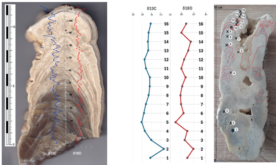
Obr. 11A. (vľavo) Pozdĺžny rez stalagmitom PS s hodnotami stabilných izotopov O a C. Čísla (čierne) predstavujú počet a poradie bodov odvŕtaných pozdĺž rezu vzorky PS s krokom 1mm. Obr. 11B. (vpravo) Pozdĺžny rez stalagmitom Benj24-1 s hodnotami stabilných izotopov O a C. Čísla (červené) predstavujú miesta odvŕtaných vzoriek na reze stalagmitu Benj24-1.
