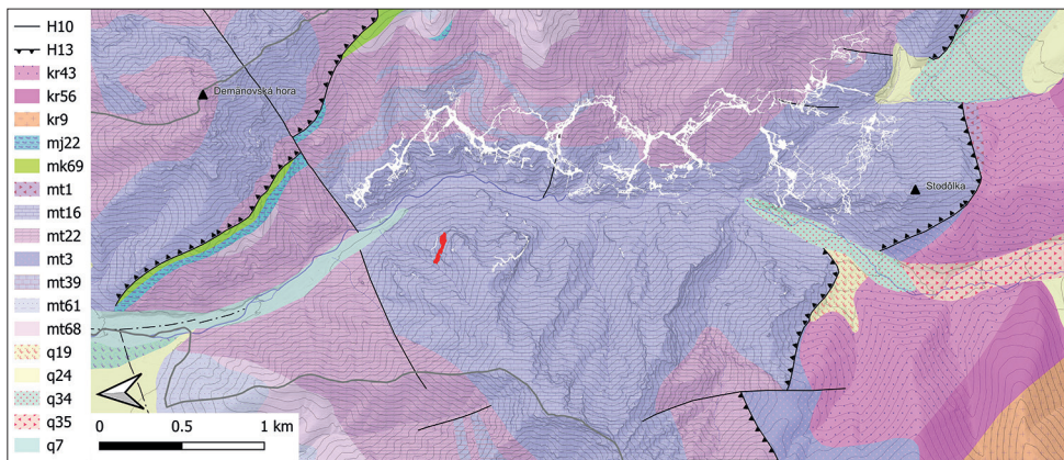
Obr. 3. Geologická mapa (podľa Biely ed., 1992) vybranej časti Demänovskej doliny s vyznačením polohy Demänovských jaskýň (bielou; podľa Herich, 2023) a Jazernej v Korenci (červenou). Vysvetlivky: H10 – zlomy, zistené, predpokladané; H13 – príkrovové línie 1. rádu, zistené; kr43 – biotitické a dvojsľudové granodiority s ružovými K-živcami (prašivský typ); kr56 – biotitické tonality až granodiority (ďumbiersky typ); kr9 – leukokratné granity; mj22 – pestrý súbor piesčitých vápencov, krinoidových a hľuznatých vápencov; mk69 – mraznické súvrstvie: sivé a tmavosivé slienité vápence (niekedy s hľuzami rohovcov), slieň, slieňovce, vápnité bridlice; mt1 – dolomity, rauvaky, brekcie, pestré vápence, žltkavé zrnité dolomity, miestami bunečné (rauvaky); mt16 – gutensteinské súvrstvie (gutensteinské vrstvy) – gutensteinské (annaberské) vápence: tmavosivé a čierne hrubolavcovité, vrstevnaté, červenkovité vápence; mt22 – ramsauské dolomity: sivé vrstevnaté dolomity; mt3 – lúžňanské súvrstvie: svetlosivé, ružové, červené kremence, kremenné pieskovce, arkóзовé pieskovce, konglomeráty; mt39 – podhradské vápence: sivé až tmavosivé vápence gutensteinského typu, lavicovité, organodetritické, krinoidové, lumachelové; mt61 – karpatský keuper: kremenné pieskovce, arkózy, zlepenec, ílovité bridlice, dolomity; mt68 – hlavné dolomity: svetlé, sivé masívne a vrstevnaté dolomity; q19 – deluviálno-polygenetické sedimenty: hlinito-ílovité a piesčité svahové hliny; q24 – deluviálne sedimenty vcelku: litofaciálne nerozlíšené svahoviny a sutiny; q34 – glacifluviálne sedimenty: hrubé, balvanovité až blokované piesčité štrky v nivách, nízkych terasách a nízkych kužeľoch; q35 – glacigénne sedimenty: štrky, balvany a bloky morén; q7 – fluválne sedimenty: litofaciálne nečlenené nivné hliny, alebo piesčité až štrkovité hliny dolinných nív a nív horských potokov.
