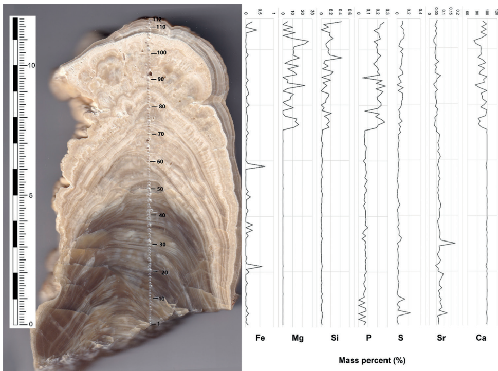
Obr. 12. Prvkové profily získané pomocou XRF pozdĺž izotopového profilu stalagmitu PS. Fig. 12. Elemental profiles obtained by XRF along the isotope profile of stalagmite PS.
