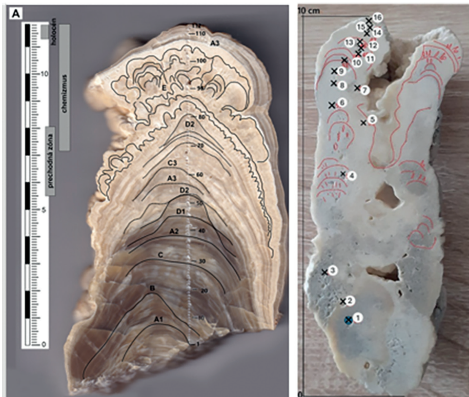
Obr. 7. Architektonické prvky piateho rádu (morfostratigrafické jednotky) znázornené písmenami A-E v pozdĺžnych rezoch obidvoch stalagmitov PS (7A) a Benj24-1(7B). 7A) Rez stalagmitom PS zobrazuje 5 morfostratigrafických jednotiek; Časť stalagmitovej sekcie tmavej farby zobrazuje štyri po sebe idúce morfostratigrafické jednotky, od základne po vrch: spodná jednotka zodpovedá typu A (A1, A2, A3) guľovité morfostratigrafické jednotky zodpovedajúce „zvonovitému“ podtypu predstavujú malú zmenu polohy bodu kvapkania navzájom, A1 a A2 sú oddelené dvoma jednotkami: B - špicatou a C - s plochým vrcholom („podtyp meseta“), nad ktorým je jednotka D - volánovitá morfostratigrafická jednotka s dobre diferencovanými centrálnymi a periférnymi časťami. Prítomné sú progradáčné a retrakčné intervaly v rámci jednotiek. Svetlú časť stalagmitového rezu nad bodom 55 po bod 80 nazývame „prechodnou zónou“, ktorá reprezentuje striedanie sa podtypov volánovitej morfostratigrafickej jednotky („vyprázané vajce“ / „mníšska hlava“). Hranice medzi po sebe idúcimi jednotkami sú retrakčné. Prechodná zóna prechádza cez rozmanité prechodné typy do E-chaotickej morfostratigrafickej jednotky (od bodu 80 do 108), ktorá je typická zložitými rastovými vzormi. Vrchol typu A3 najpravdepodobnejšie holocénneho veku má nepravidelnú topografiu povrchu, ale na jeho jednej strane (vpravo na obrázku) má pravidelne zhrubnutú narastajúcu sintrovú vrstvu z cyklicky sa opakujúcich kompaktných vrstiev kalcitu. Príčinou prudkej zmeny narastania môže byť naklonenie stalagmitu. Náhle zmeny stratigrafických vzorov môžu predstavovať časové rozpätia s rôznym trvaním. 7B) Rez stalagmitom Benj24-1 predstavuje chaotickú morfostratigrafickú jednotku, rez dokumentuje výrazne nepravidelný rast charakterizovaný chaotickým striedaním tmavších a svetlejších zón, reprezentujúcich kompaktný (tmavší) a pórovitý (svetlejší) materiál, všadeprítomné rozpúšťacie procesy sú zreteľne vyvinuté a v centrálnej časti stalagmitu vedú k vzniku rozsiahlych dutín.
