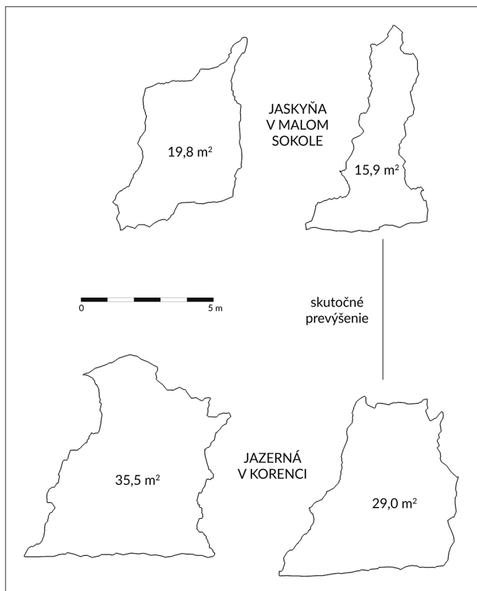
Obr. 6. Charakteristické priečne profily Jazernej v Korenci a Jaskyne v Malom Sokole. Dimenzie profilov a ich vzájomná výšková poloha sú v mierke.
