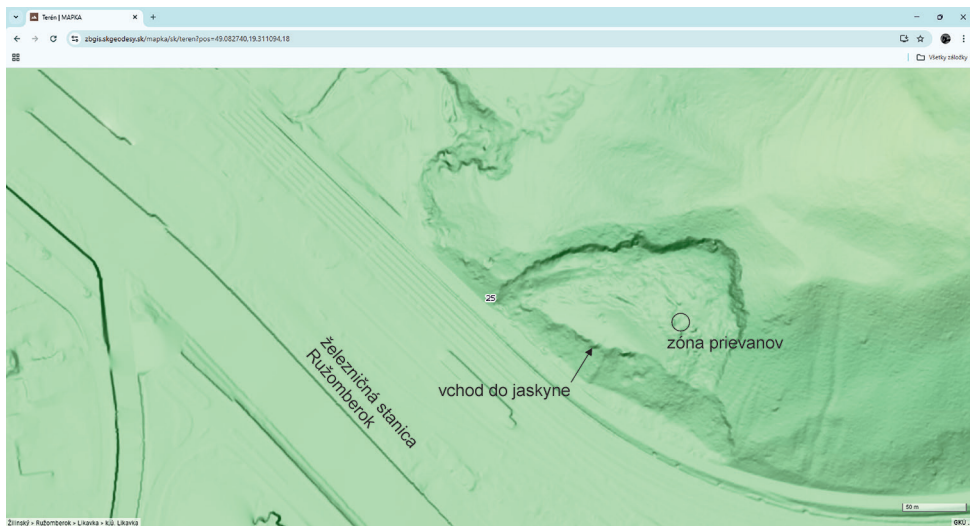
Obr. 1. Lidarová snímka zosuvu z Mnícha s vyznačením polohy jaskyne a odtopených miest v snehu.
